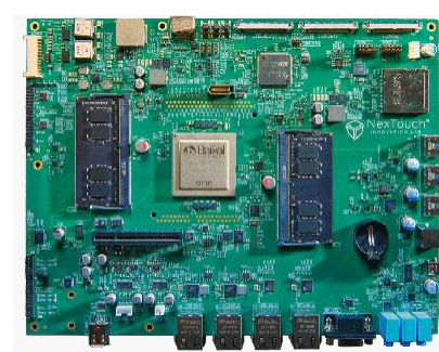
Управляющие платы на российских процессорах
